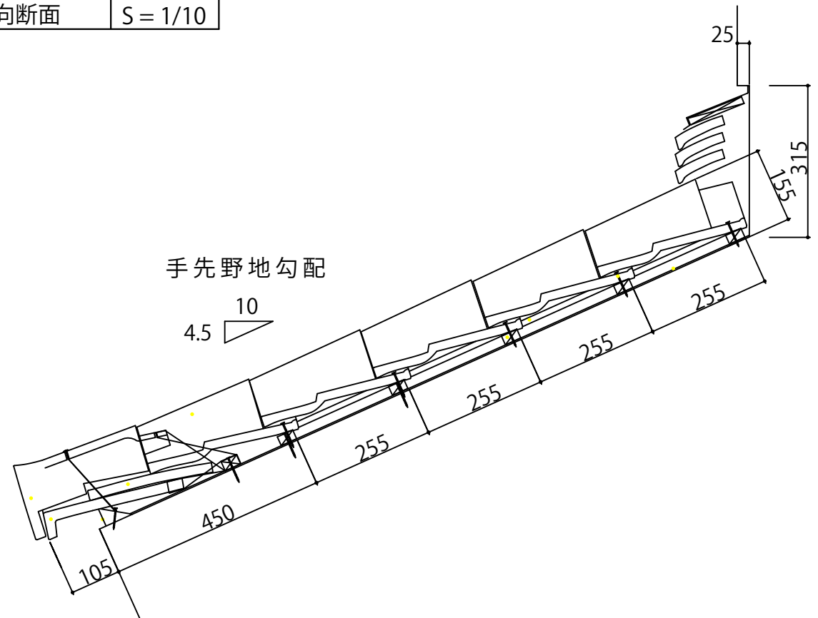
軒積断面 S = 1/10
