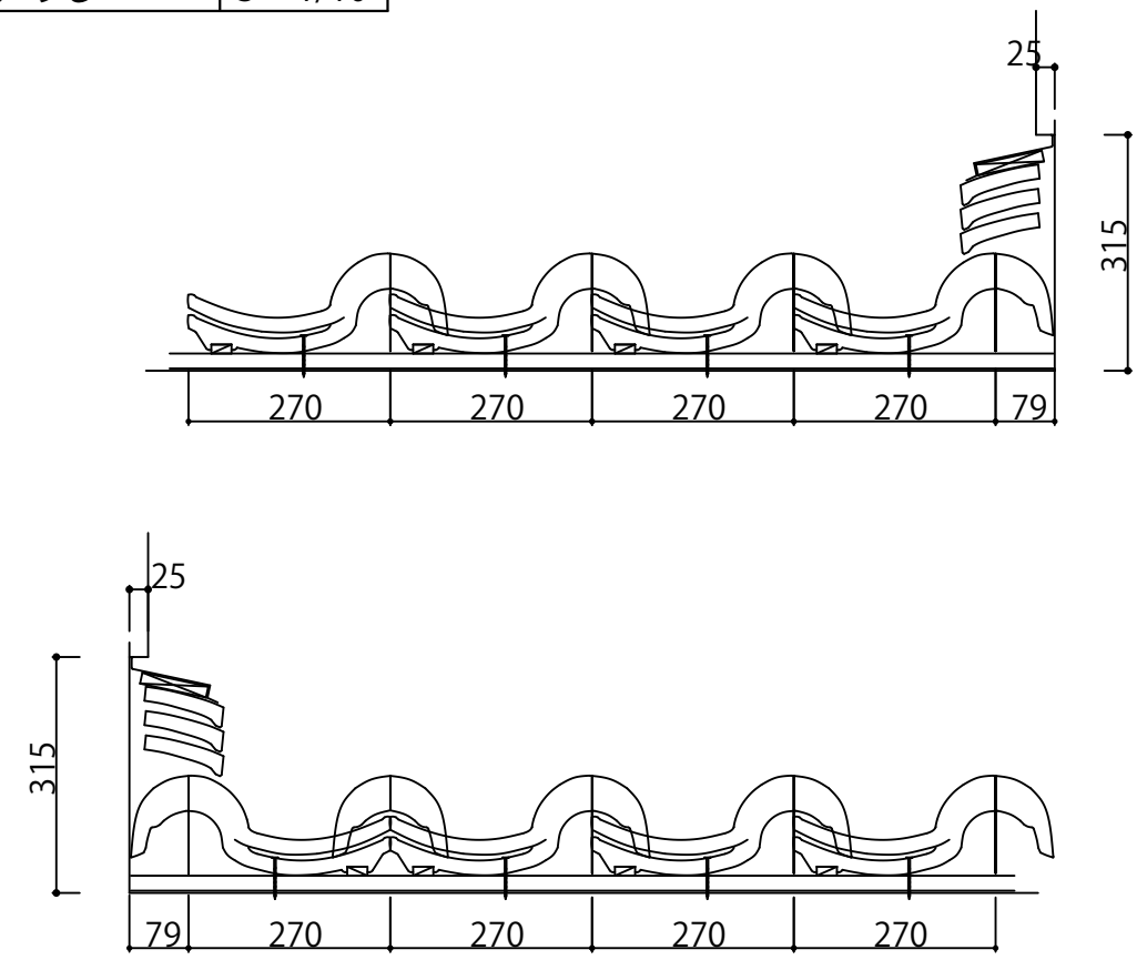
壁際付けのし S = 1/10
